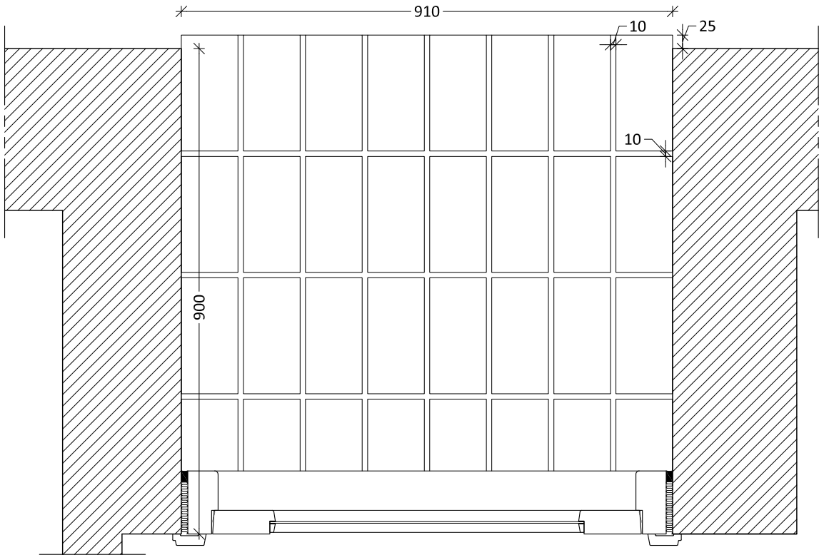
Belægninger i hoveddørsniche Mål 1:10
